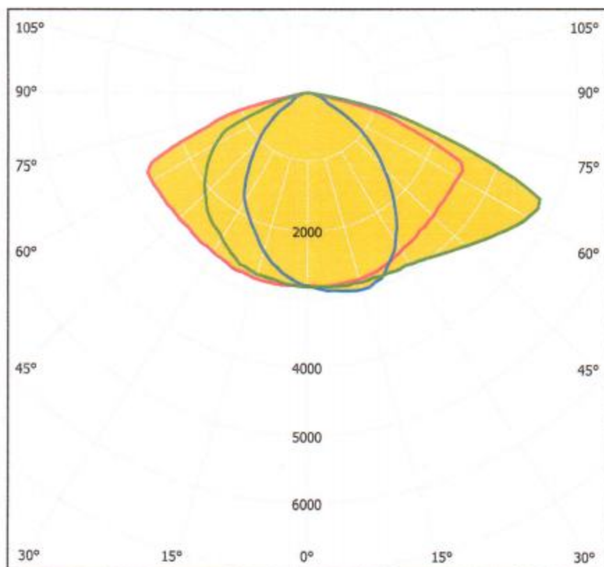
Рисунок 1 – КСС образца светильник светодиодный ДКУ-01-064-5КК-10900-Ш-IP67 в поперечной (C0-C180) (красная кривая), продольной (C90-C270) (синяя кривая) плоскостях и плоскости максимальной силы света (C164-C344) (зеленая кривая)
