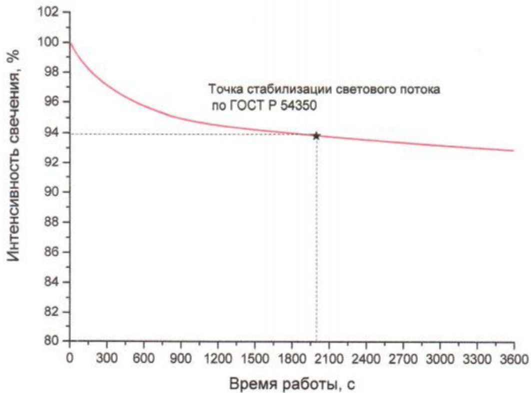
Рисунок 3 – График стабилизации светового потока образца светильник светодиодный ДКУ-01-064-5КК-10900-Ш-IP67
