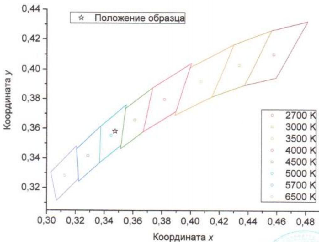
Рисунок 4 – Положение образца на диаграмме цветности МКО 1931г. и области допустимых значений номинальной КЦТ по ГОСТ Р 54350-2015
