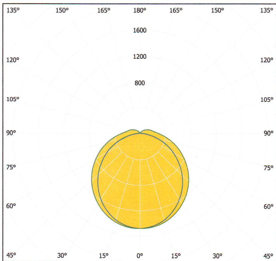
Рисунок 1 – КСС образца светильник светодиодный ДСП-03-036-5KK-4250-Д120-IP66 в поперечной (C0-C180) (красная кривая), продольной (C90-C270) (синяя кривая) плоскостях и плоскости максимальной силы света (C0-C180) (зеленая кривая)
