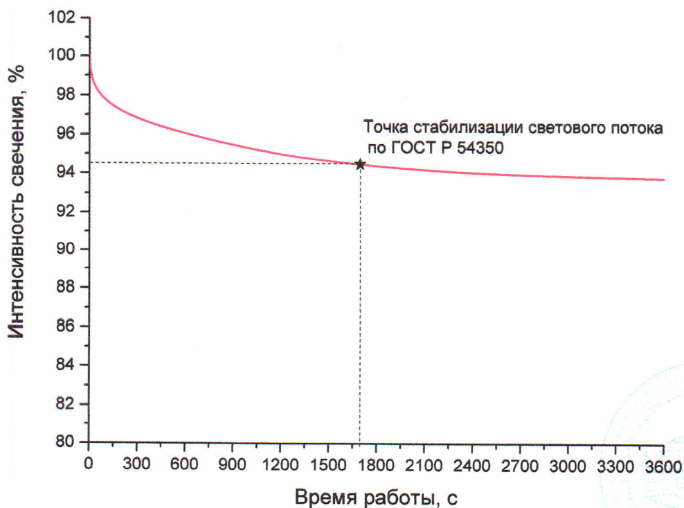
Рисунок 2 – График стабилизации светового потока образца светильник светодиодный ДСП-03-036-5KK-4250-Д120-IP66
